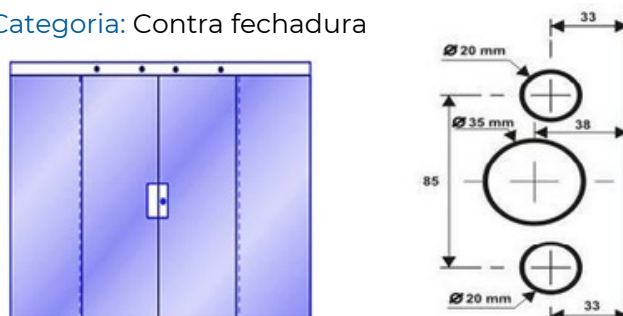
S3211 - Contra fechadura com aba de proteção
