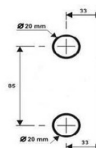
S3230 - Testeira da fechadura para alvenaria
