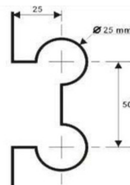
1306 - Suporte para união de 2 vidros com pino
