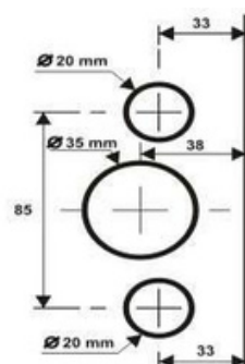
S3530 - Contra fechadura para janela de correr
