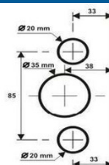
S3530 - Fechadura para porta de correr
