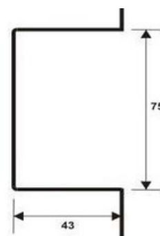
1523 - Trinco com mola para basculante central
