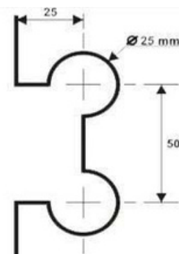
1231 - Dobradiça bucha para basculante
