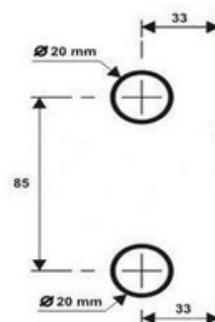
S3536 - Contra fechadura para janela de correr
