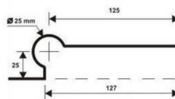
1504A - Batedeira em alvenaria para 1520
