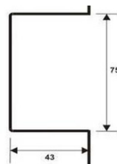
S1801 - Batedeira para trinco de basculante
