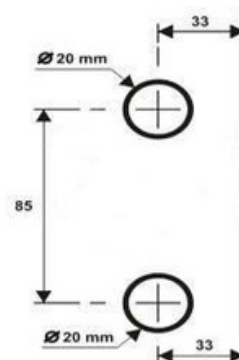
S3230 - Testeira da fechadura para alvenaria
