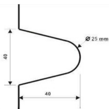
1230 - Dobradiça bucha para basculante
