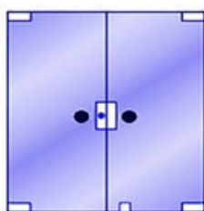
1523 - Trinco com mola para basculante central
