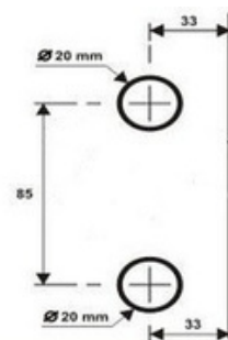
1571G - Bate-fecha para janela grande com furação * sem miolo*
