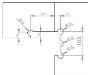
1209G - Facão grande lateral e bandeira
