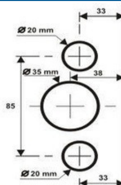
1510XJ - Fechadura para janela de correr
