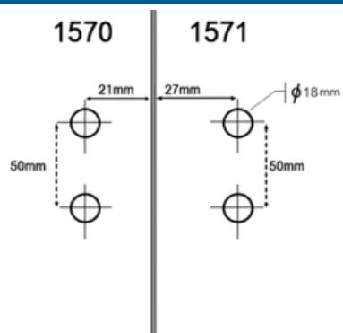
V1570 90° - Bate-fecha de canto 90° V/V
