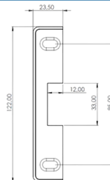
1511AXPU-Testeira p/ 1510XC perfil U maior
