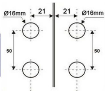
V1570 - Bate-fecha central V/V modelo Vialtec com tranca
