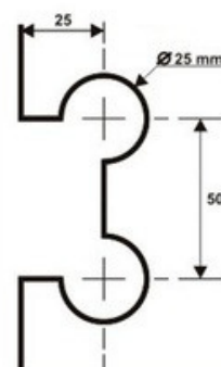
1231 - Dobradiça bucha para basculante 100 x 50 mm
