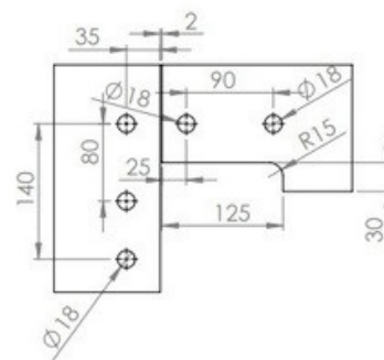
1209PG - Facão grande lateral para bandeira
