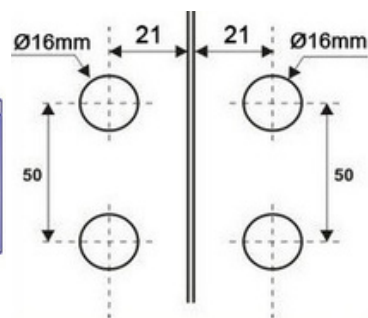
1570NCAD - Bate-fecha central com porta cadeado V/V
