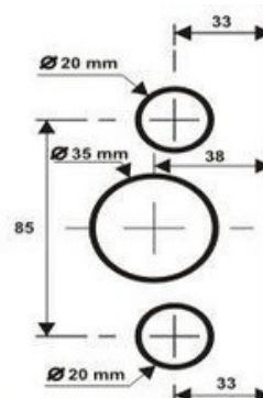
V1510X - Fechadura para porta de correr modelo Vialtec
