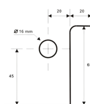
1810 D - Trinco direito para janela de correr
