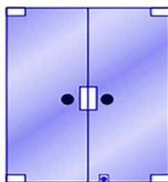
1201 - Pivô para dobradiça 1101, 1123, 1130 e 1101R
