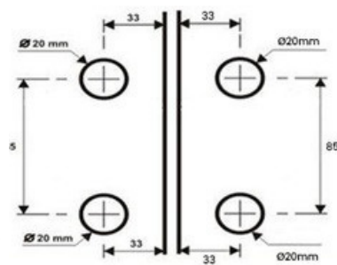
V1570 - Bate-fecha central V/V modelo Vialtec com tranca
